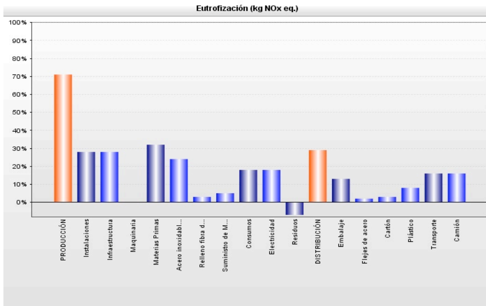
Eutrofizazioa adierazlearen arabeko ingurumen-alderdiak
